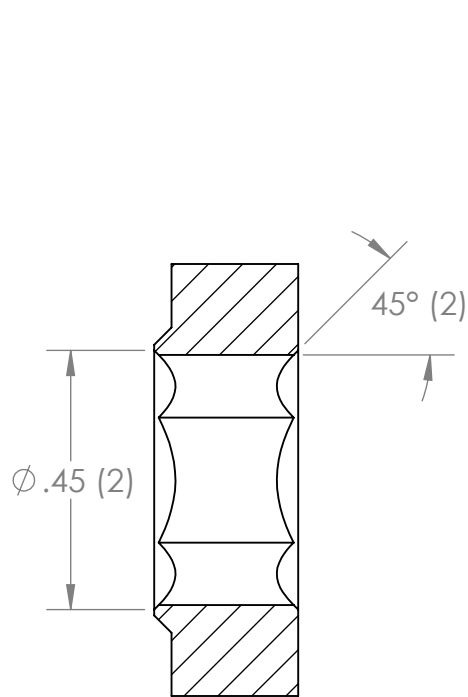
SECTION A-A
